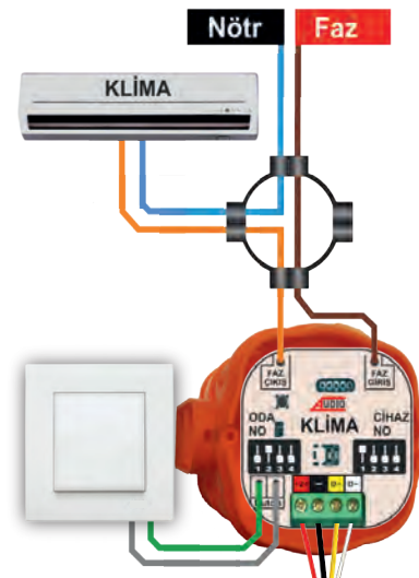
OTOMASYON KABLOSU(OK-4)
