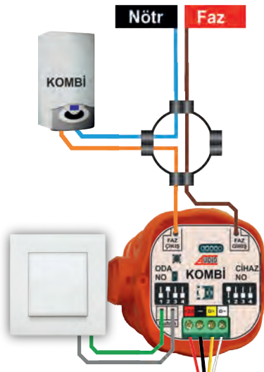
KOMBİ BAĞLANTISI
